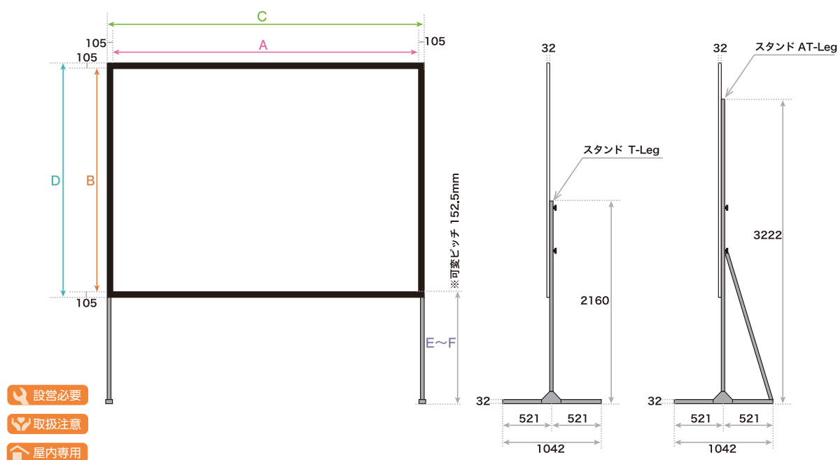
89-1 16:9 100~275インチフロントスクリーン
