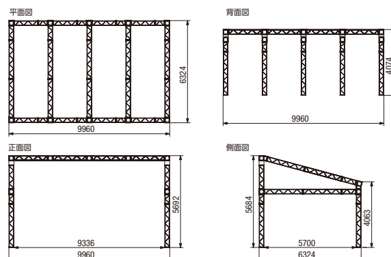
■3K×5K 外形図
