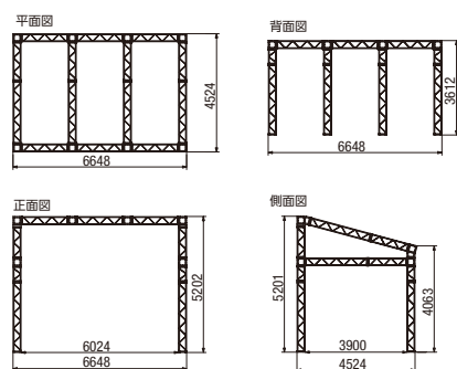
■2K×3K 外形図
